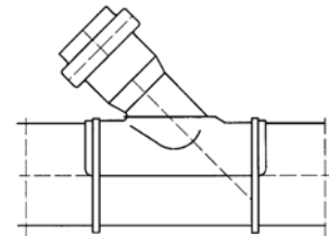
Bild 15 Klebschelle
